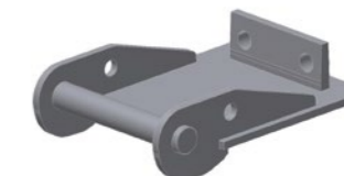
Adapterplatte SWE-KSW-010LA
